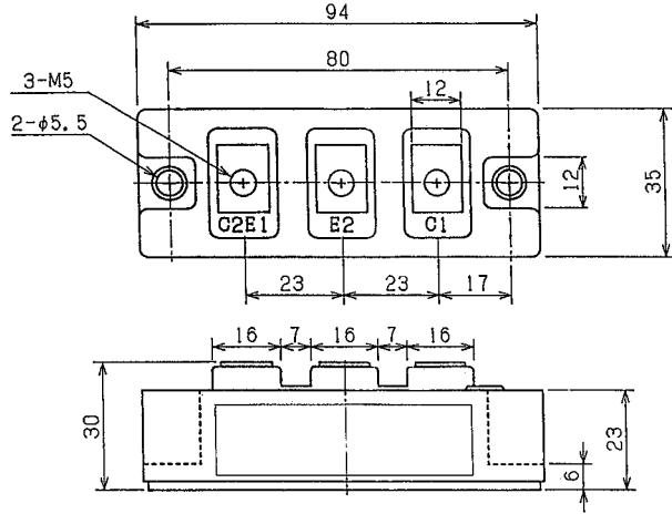
外形寸法図 OUTLINE DRAWING (単位 Dimension : mm)
